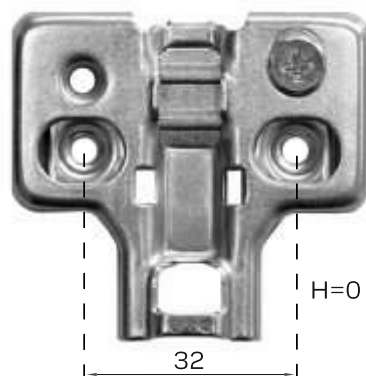
МОНТАЖНАЯ ПЛАНКА
