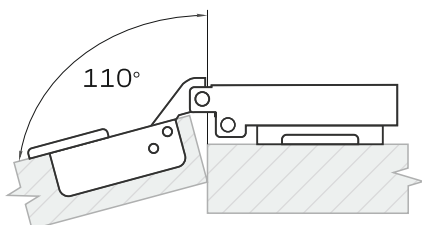
ПОЛУНАКЛАДНАЯ
