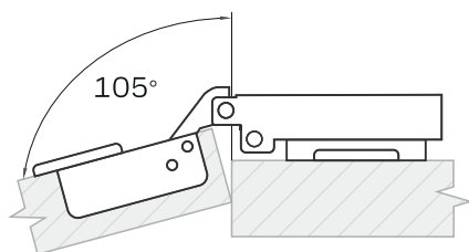
ПОЛУНАКЛАДНАЯ
