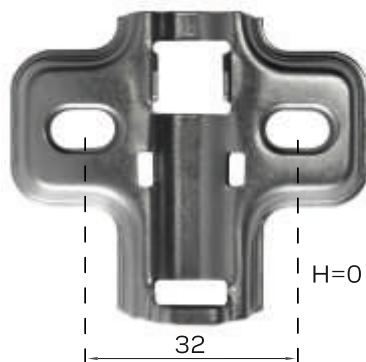
ВКЛАДНАЯ
