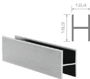
ПРОФИЛЬ ГОРИЗОНТАЛЬНЫЙ СРЕДНИЙ ЛАЙТ (БЕЗ ВИНТА)
